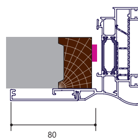
Fig 3. Moulure(s) intérieure(s) rapportée(s) (option)
