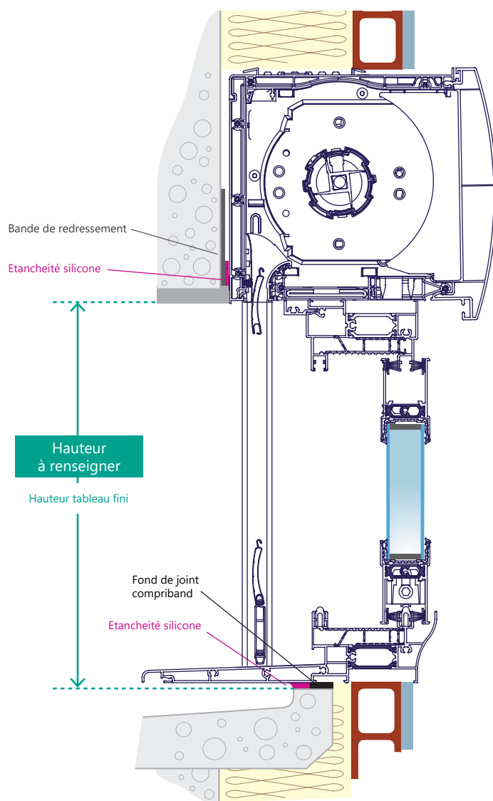
Fig 13. Coupe verticale
