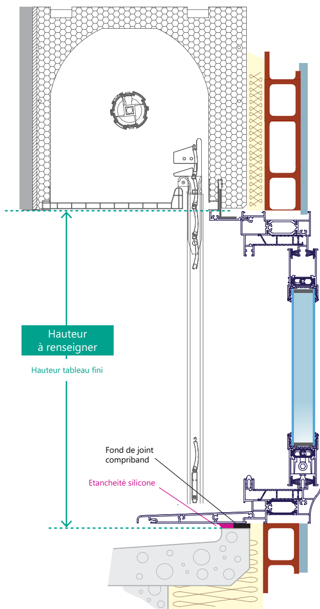
Fig 16. Coupe verticale
