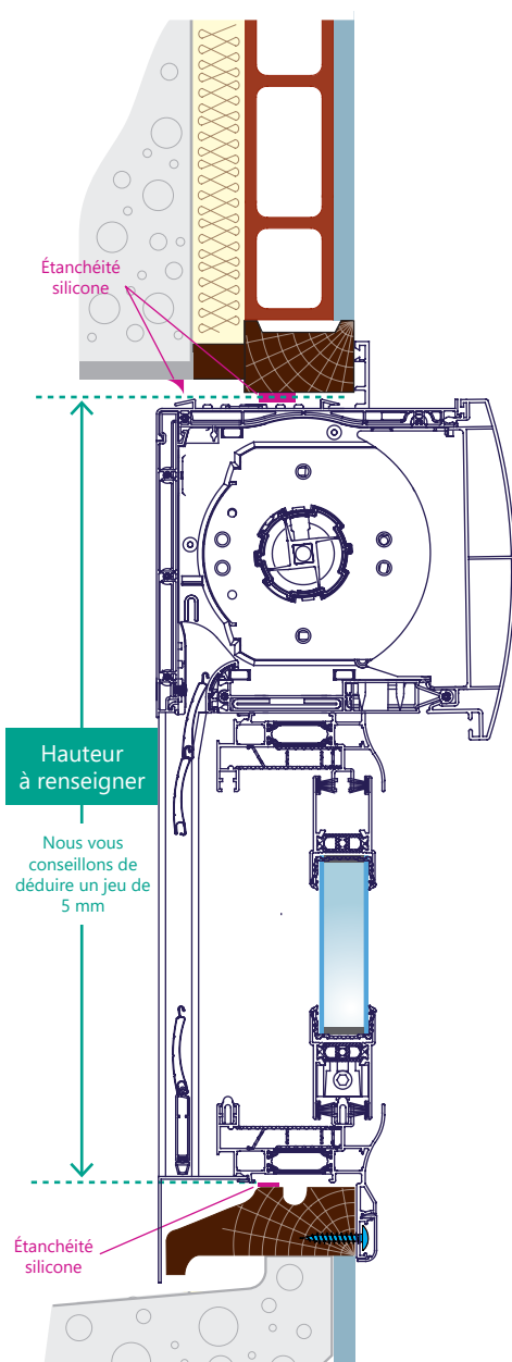
Fig 6. Coupe verticale conservation du dormant bois
