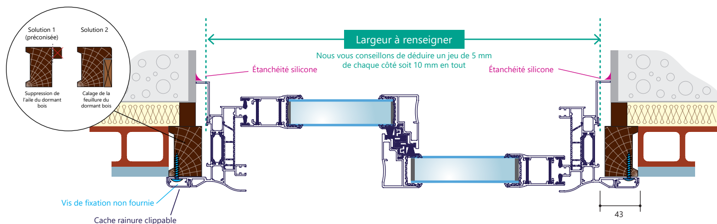
Fig 1. Coupe horizontale
