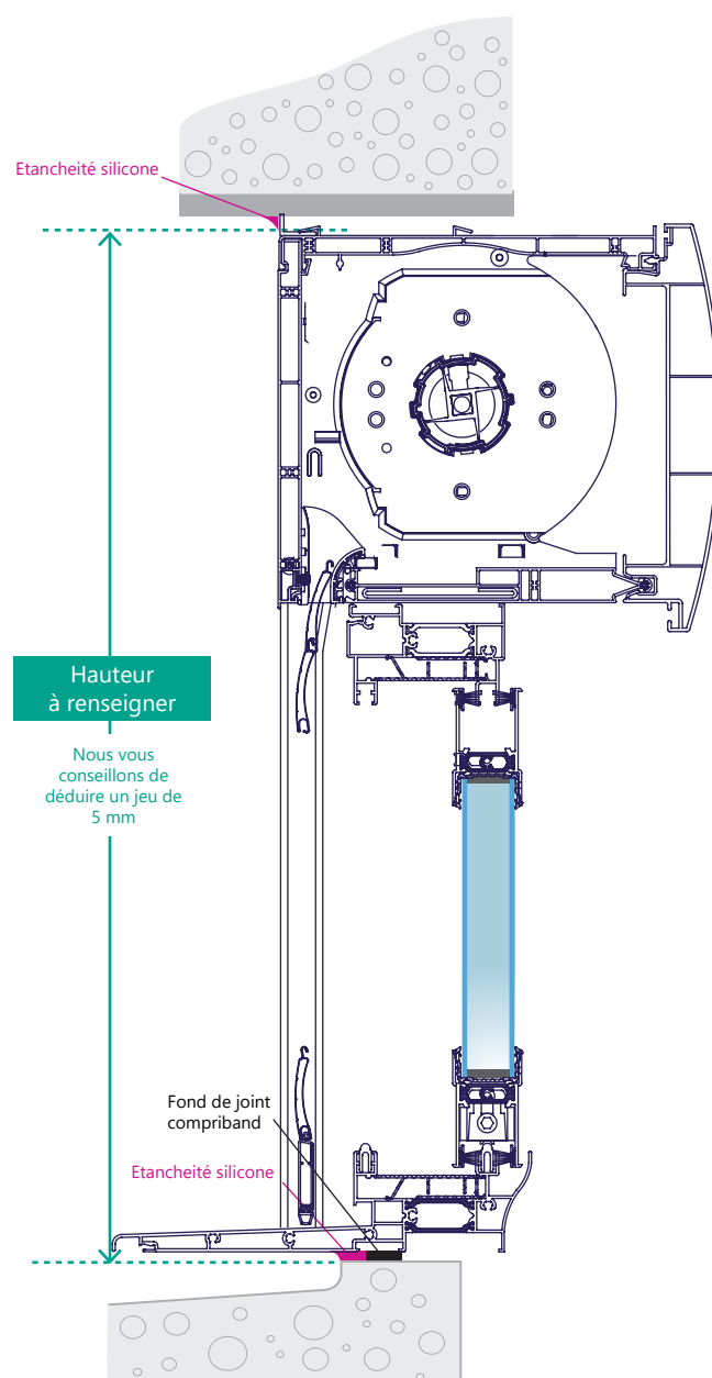
Fig 20. Coupe verticale avec volet roulant
