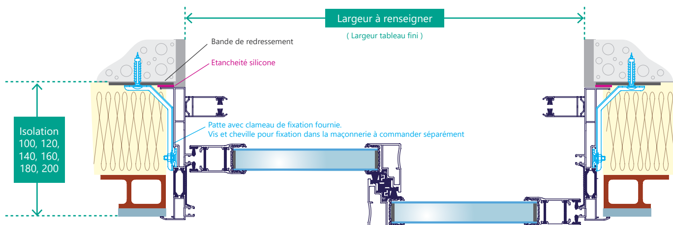
Fig 15. Coupe horizontale
