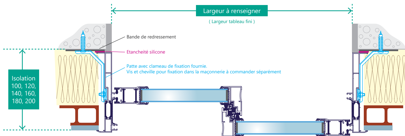
Fig 9. Coupe horizontale
