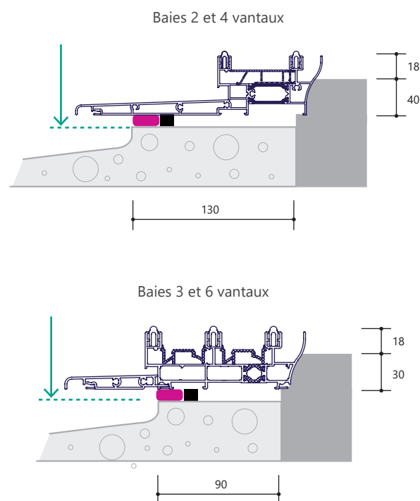
Fig 14. Seuil encastré
