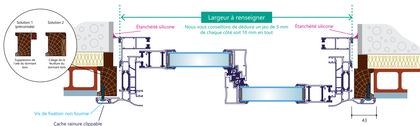
Fig 5. Coupe horizontale
