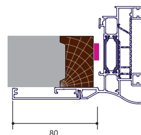
Fig 8. Moulure(s) intérieure(s) rapportée(s) (option)
