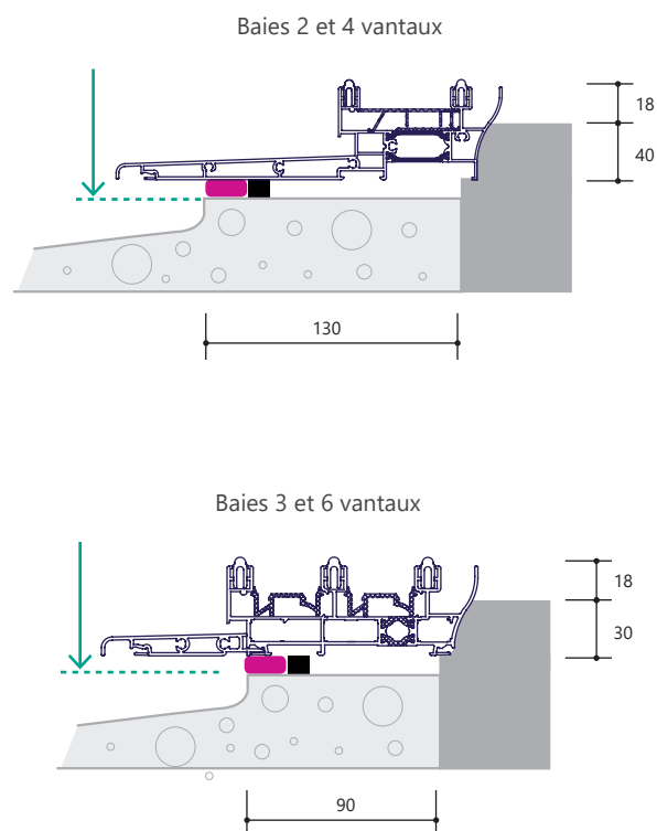
Fig 17. Seuil encastré
