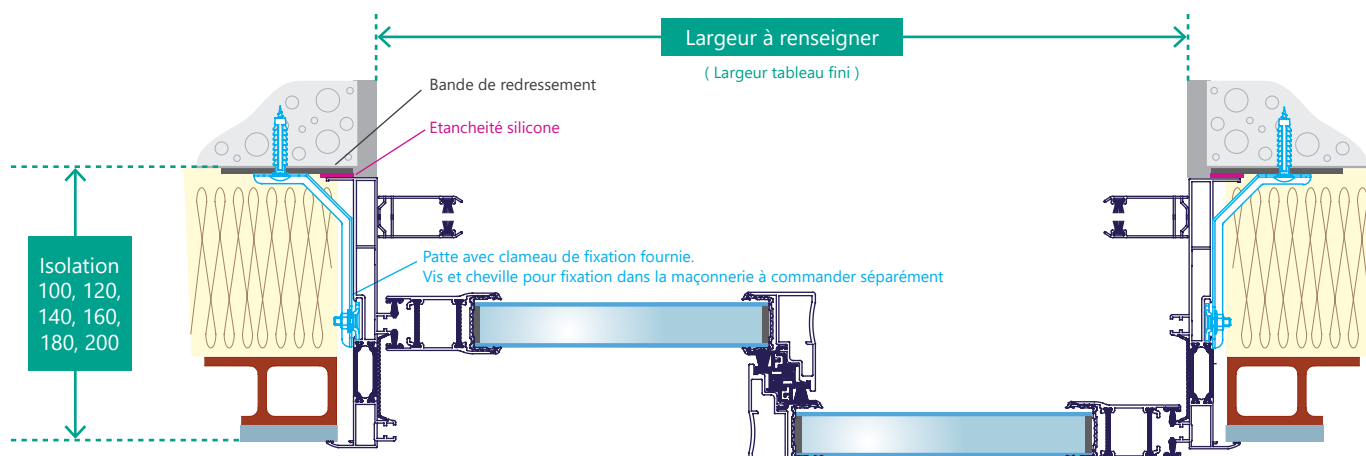
Fig 12. Coupe horizontale
